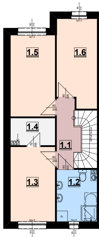
RZUT PIĘTRA-BUDYNEK 1B-lokal A
